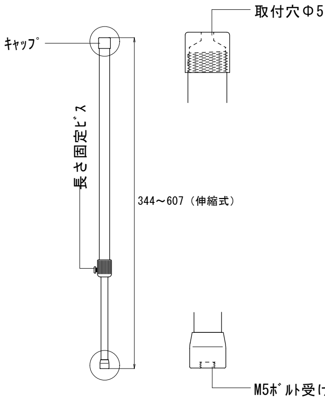
吊钩 全体图
